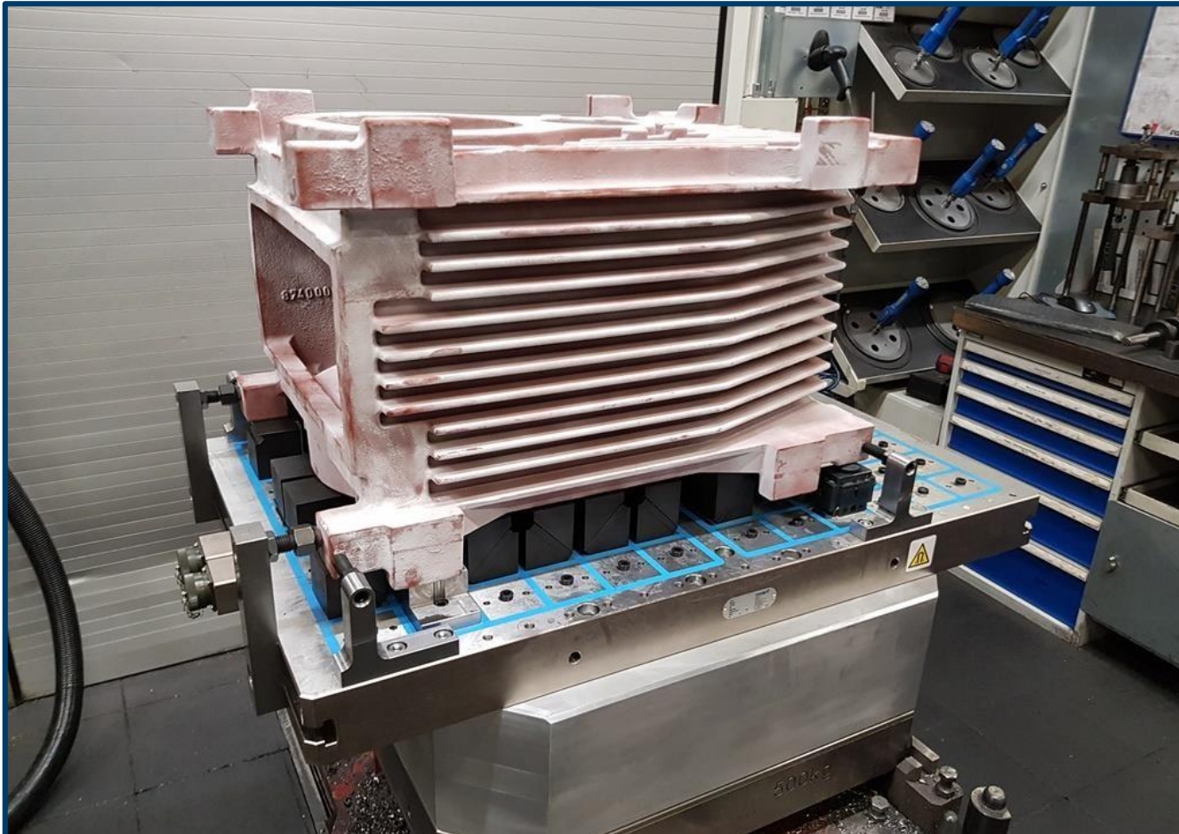
OP10 MAGNOS; fixação nas nervuras e encostos mecânicos adicionais
