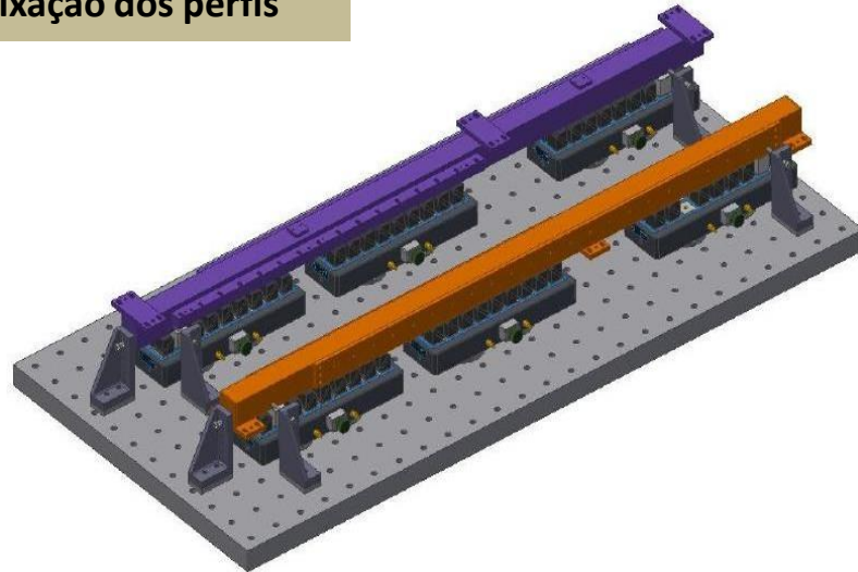
Fixação dos perfis
