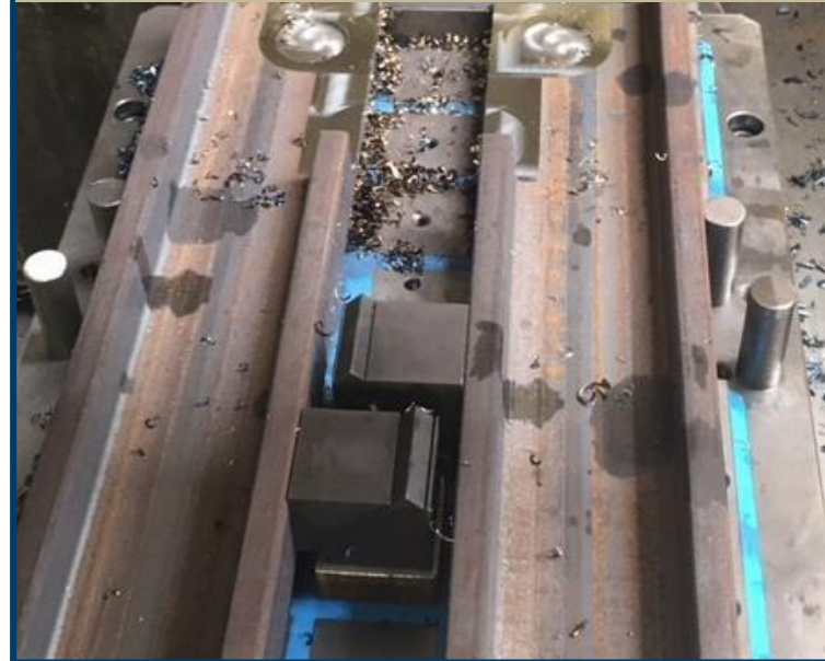
Encostos verticais para troca rápida do PV
